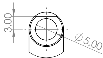
DÉTAIL B Echelle 2 : 1
