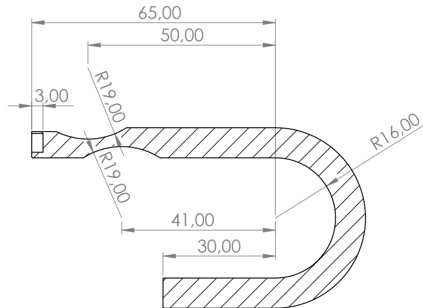
COUPE A-A
