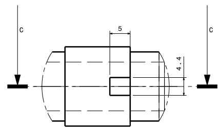
Détail B Echelle : 3:1
