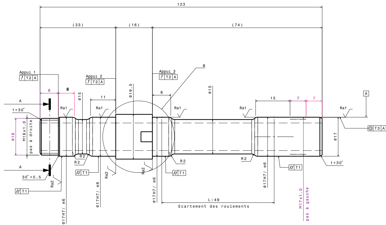
Vue de face Echelle : 3:1
