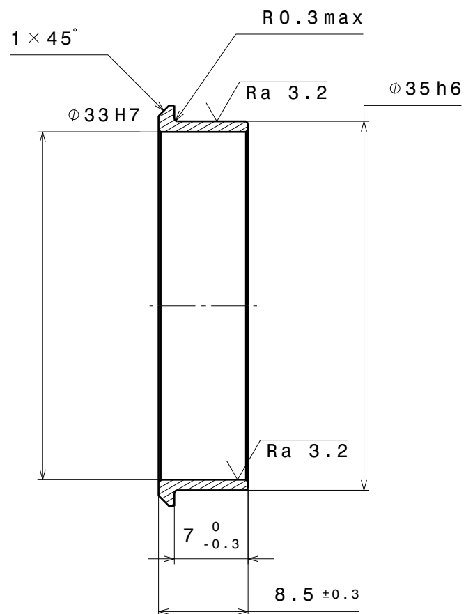
Coupe A - A 2:1
