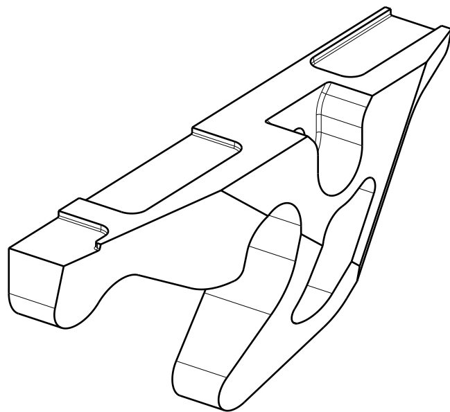
Vue isométrique Echelle : 2:3 24-2022-010A MAIN LEVAGE DROIT 2022
