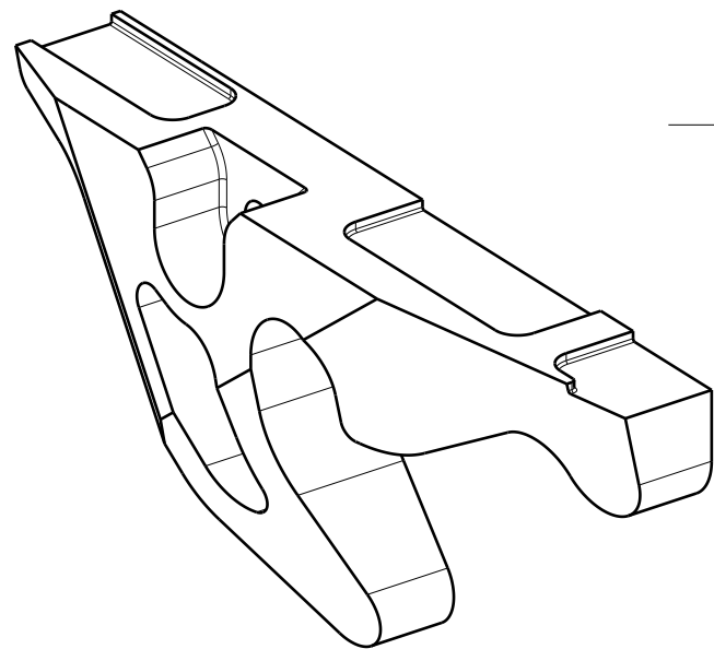
Vue isométrique Echelle : 2:3 24-2022-009A MAIN LEVAGE GAUCHE 2022
