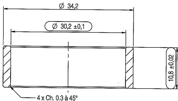
COUPE A-A
