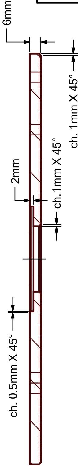
COUPE B-B
