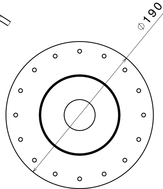
Front view Scale: 1:3
