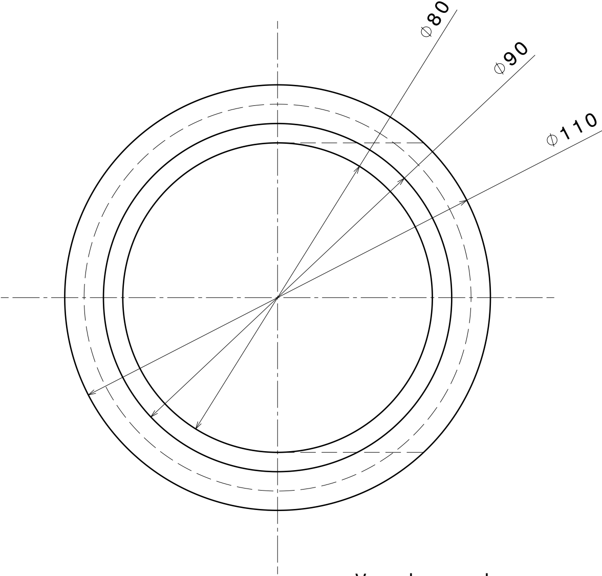
Vue de gauche Echelle : 1:1
