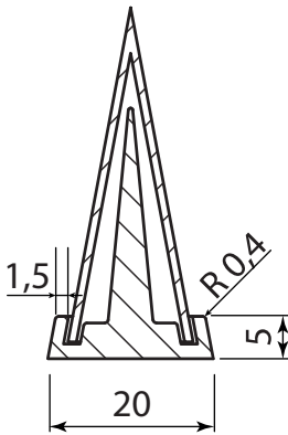
A-A (1:1)
