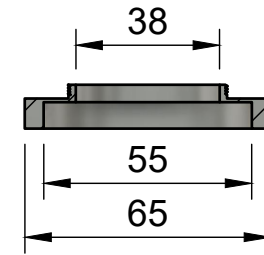
B-B (1:2)
