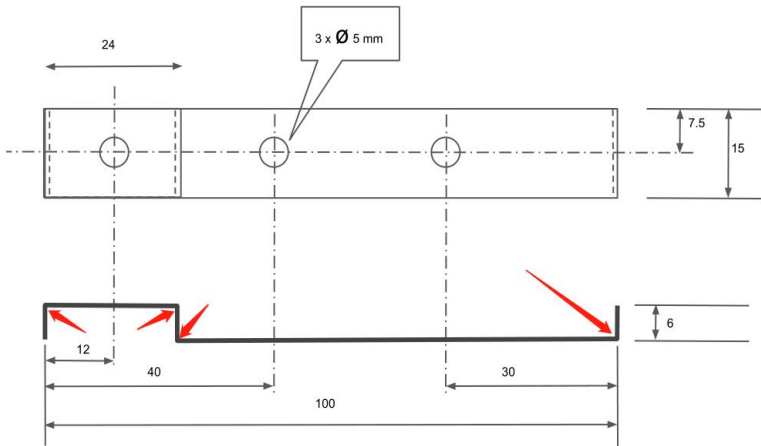
Acier Zingué Épaisseur / Galvanized Steel Thickness 1 mm
