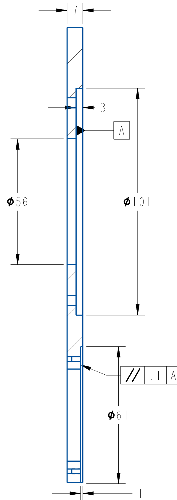
COUPE A-A
