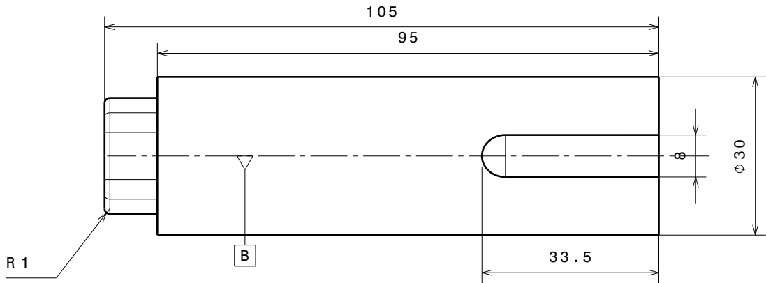
Vue de face Echelle : 1:1
