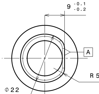
Vue de gauche Echelle : 1:1
