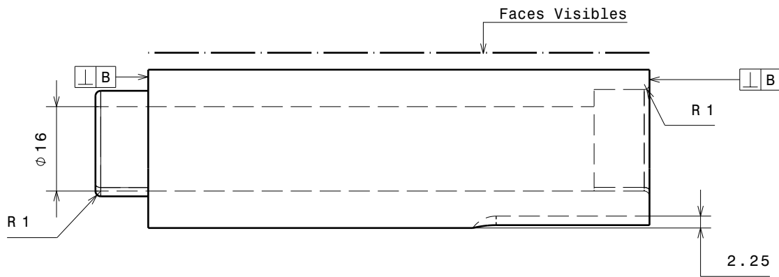
Vue de dessus Echelle : 1:1
