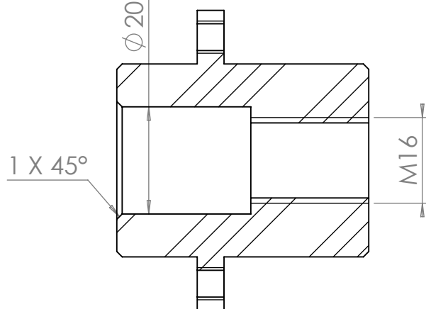
COUPE A-A
