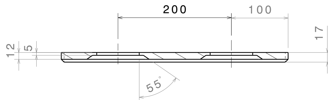
Coupe B-B Echelle : 1:4
