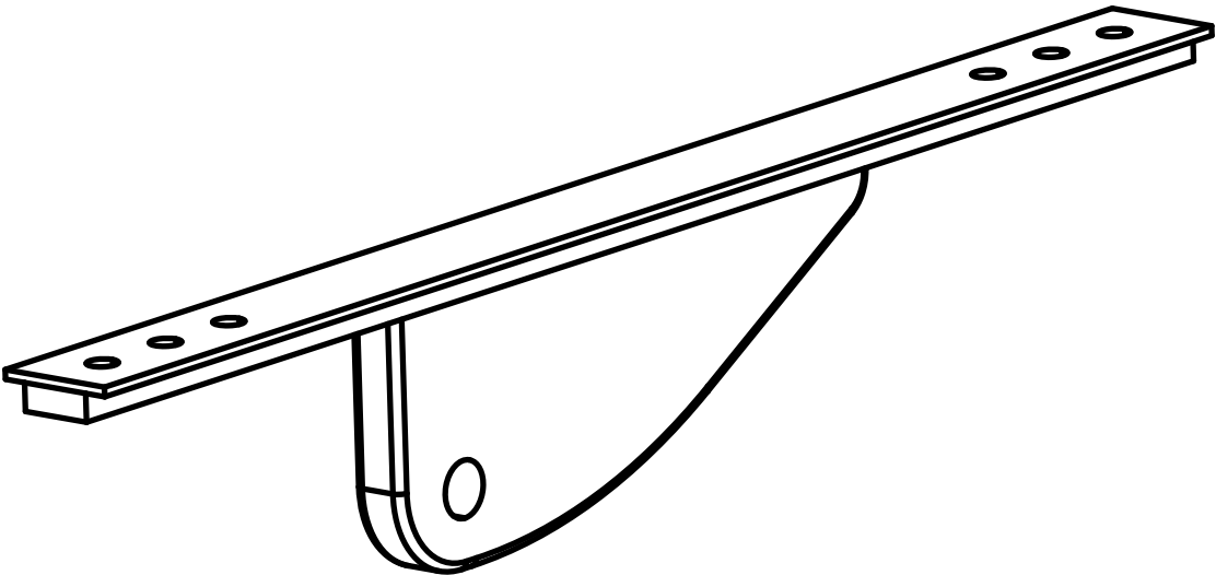
Perspective (échelle 3:5)
