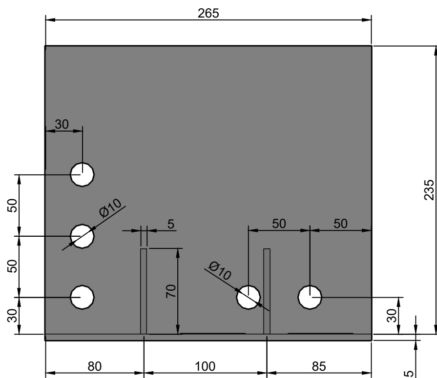
Support GAUCHE - VUE DESSUS
