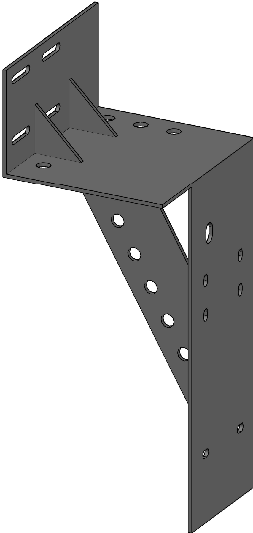
Support GAUCHE - PERSPECTIVE DESSUS ARRIERE
