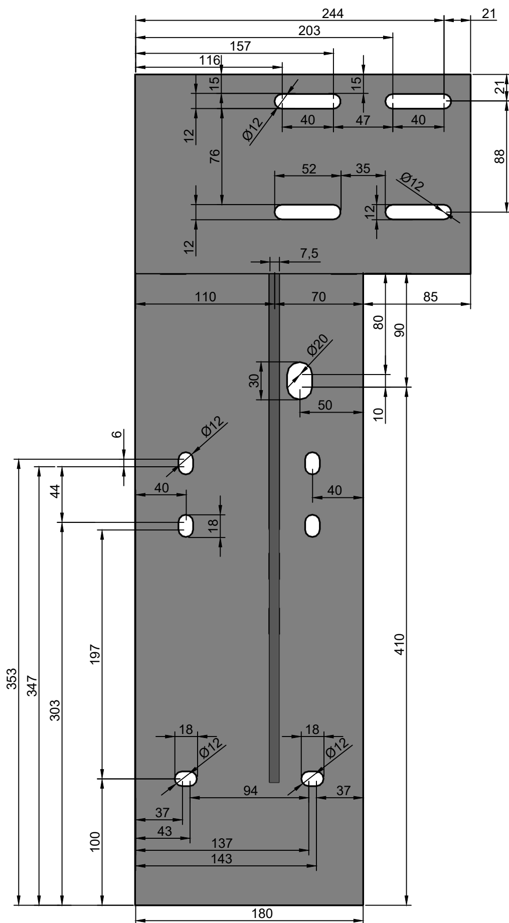
Support GAUCHE - VUE DE FACE
