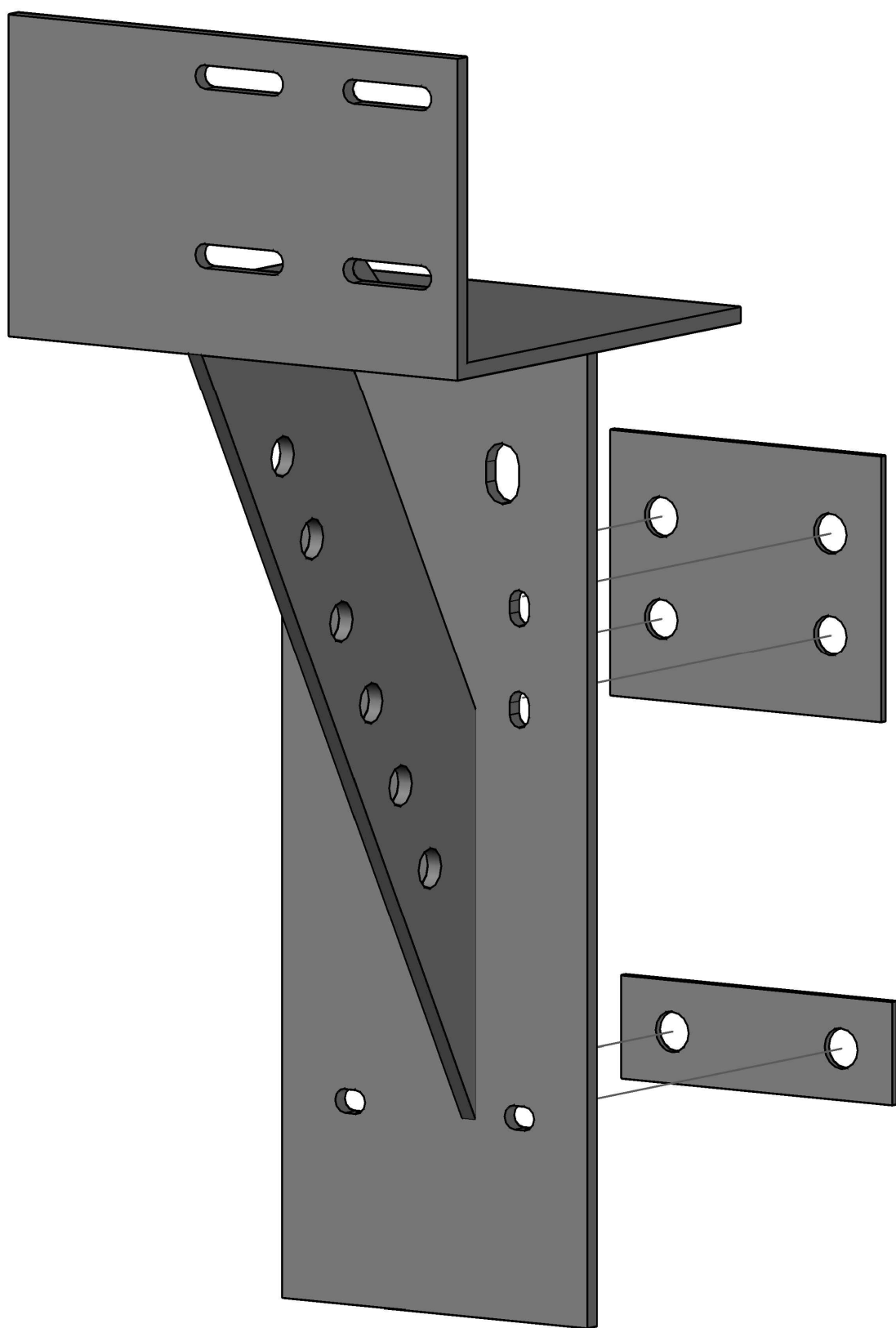
Support GAUCHE - PERSPECTIVE FACE
