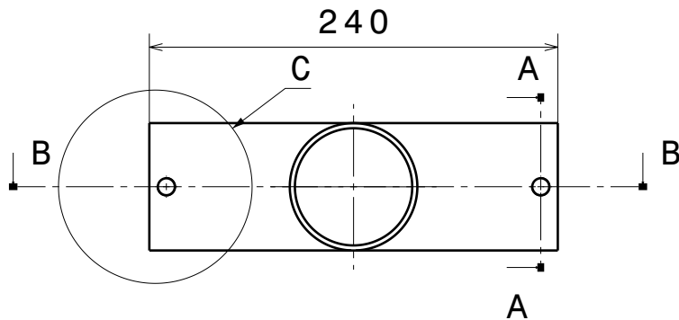
Vue de face Echelle : 1:4
