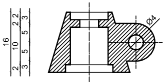
Coupe AA Ech 1/1
