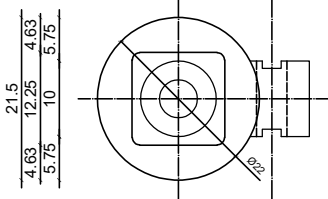
Plan Ech 1/1 - Vue de dessous
