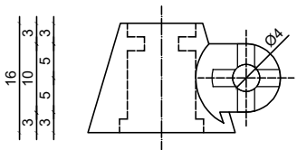
Elevation AA Ech 1/1 - Vue de côté
