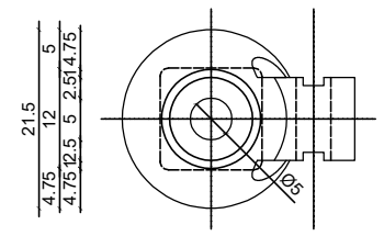
Plan Ech 1/1 - Vue de dessus
