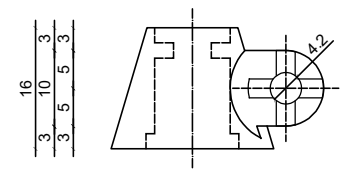
Elevation AA Ech 1/1 - Vue de côté
