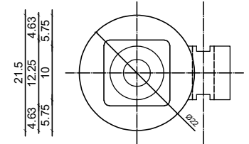
Plan Ech 1/1 - Vue de dessous
