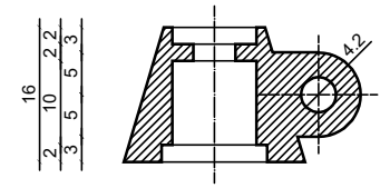
Coupe AA Ech 1/1
