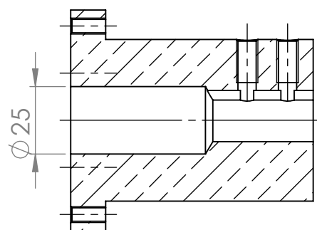
COUPE A-A
