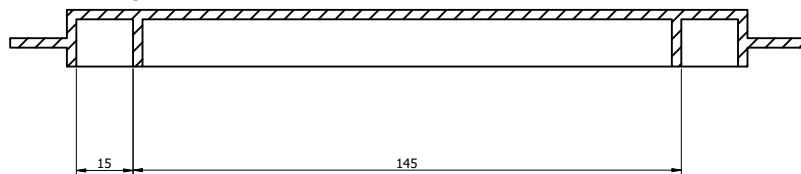
Coupe B:B
