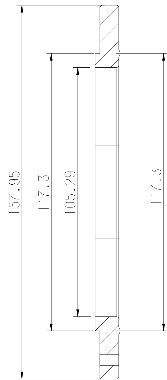
COUPE B-B
