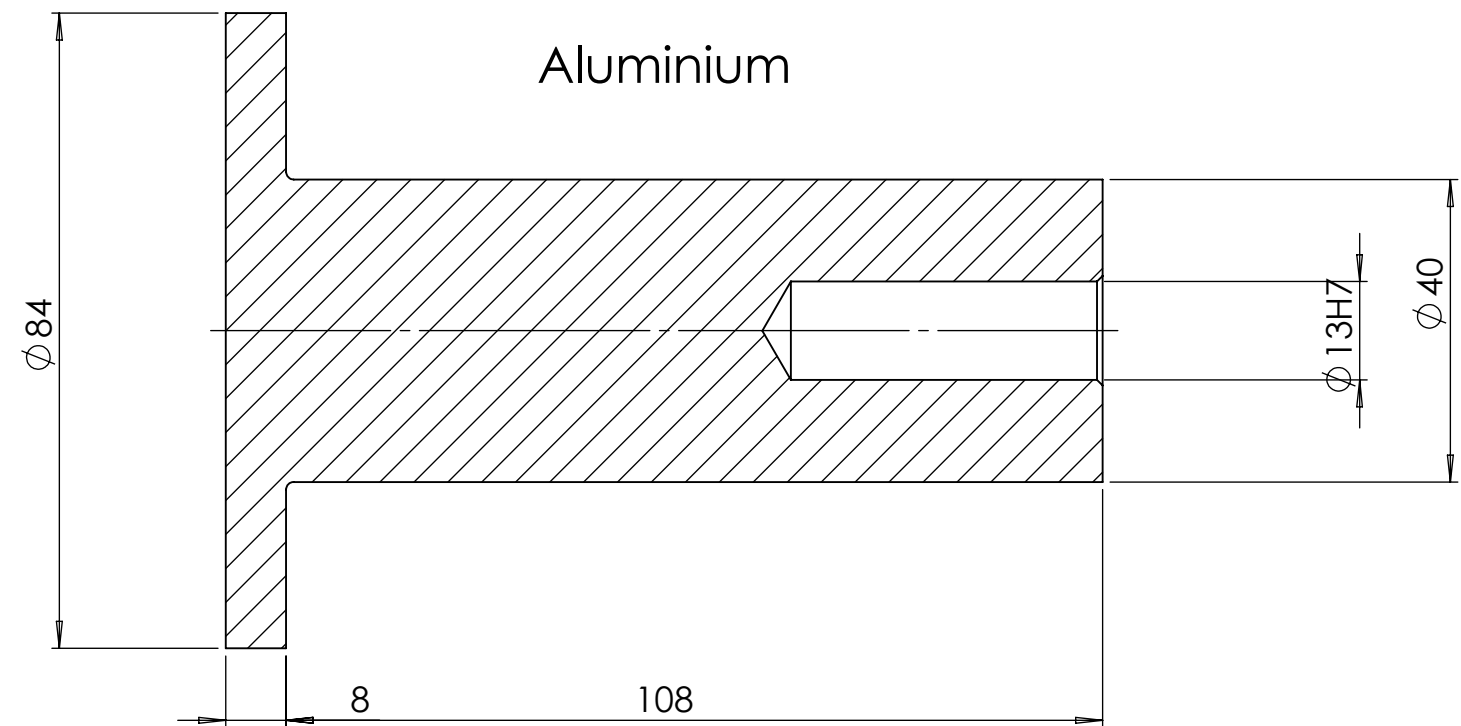
COUPE B-B
