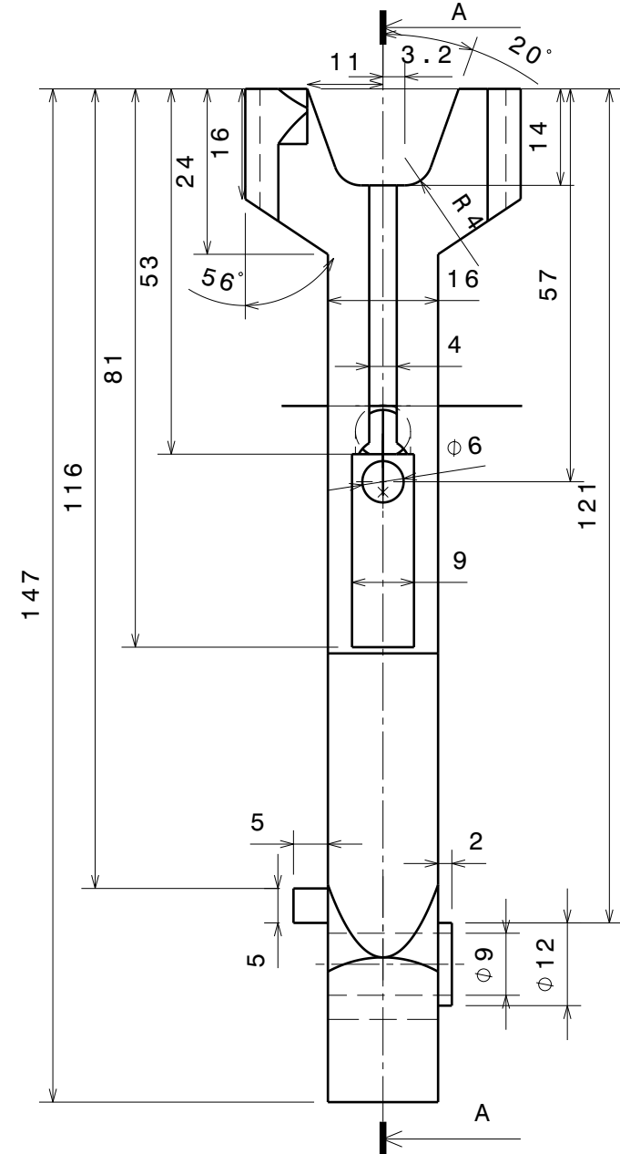
Vue de face Echelle : 1:1
