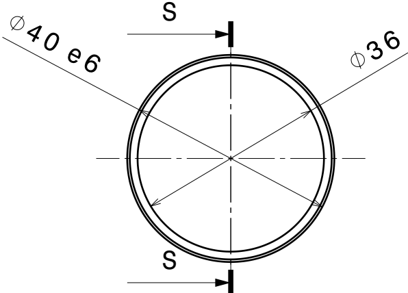
Entretoise moyeu Echelle : 1:1
