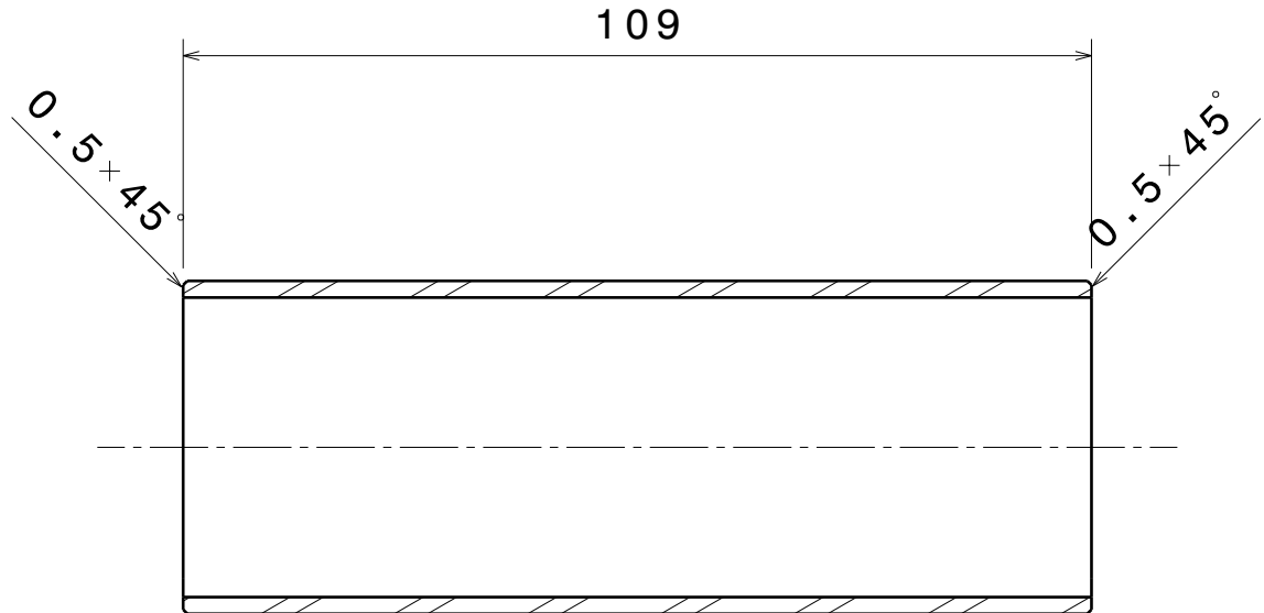
Coupe S-S Echelle : 1:1
