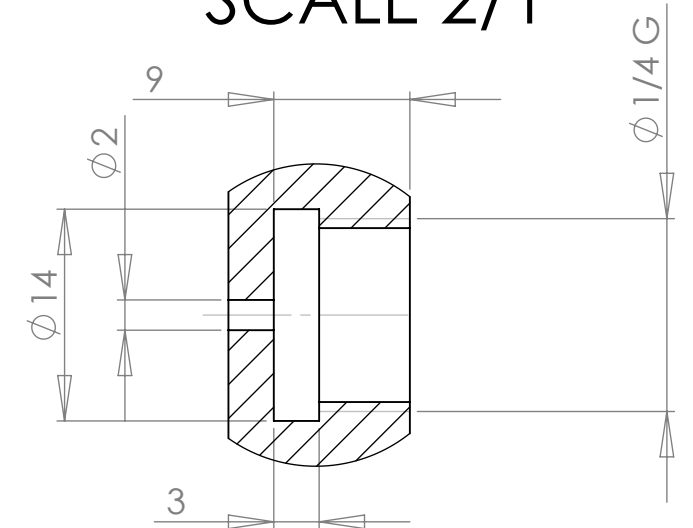
DÉTAIL C ECHELLE 2 : 1 SCALE 2/1
