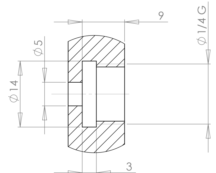
DÉTAIL C ECHELLE 2 : 1 SCALE 2/1
