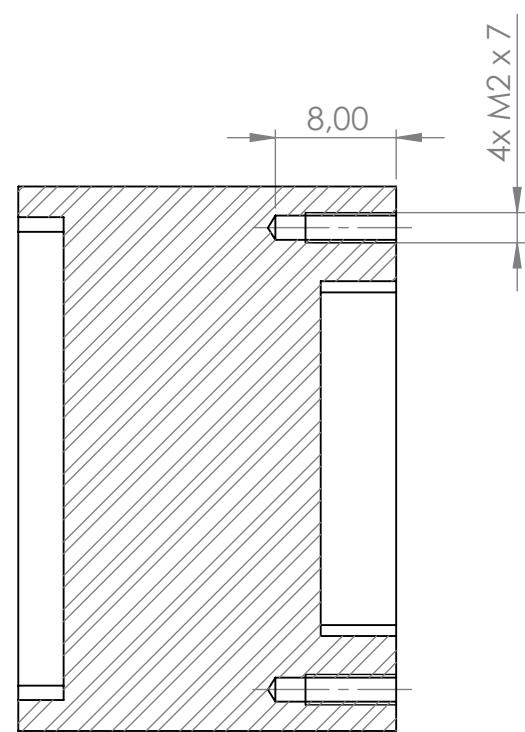
COUPE C-C
