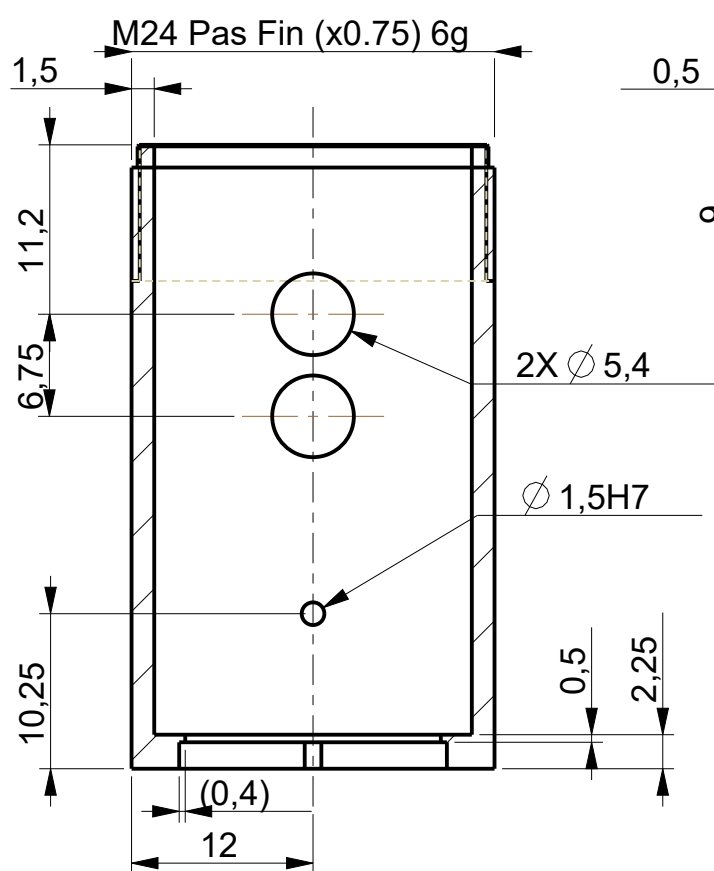
COUPE A-A
