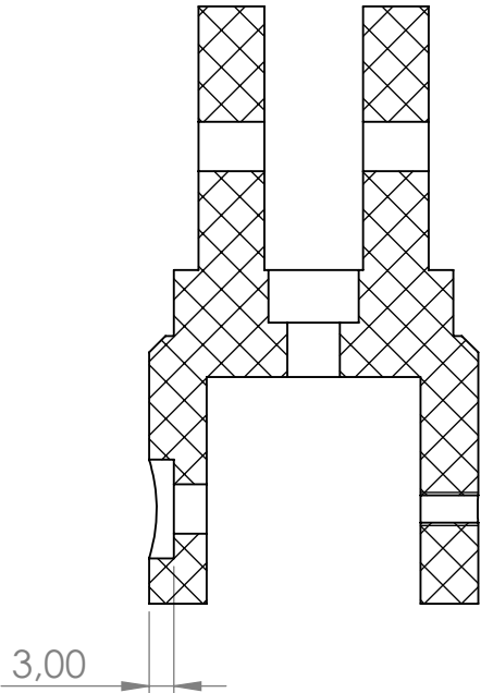
COUPE A-A
