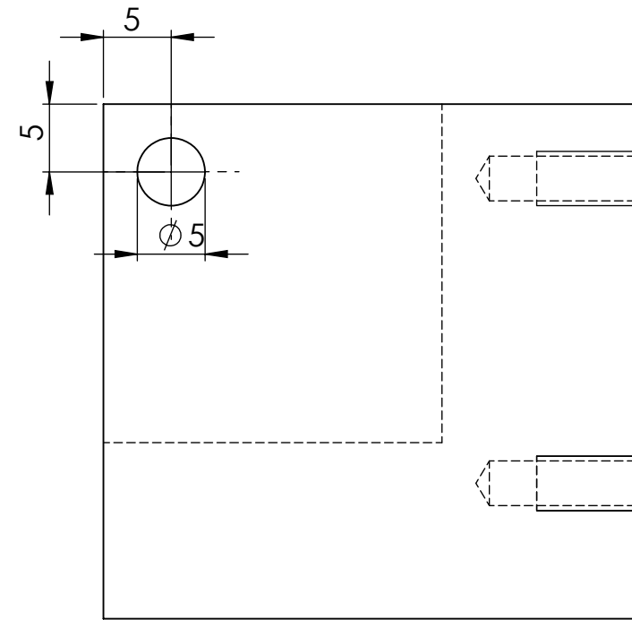
Vue Droite
