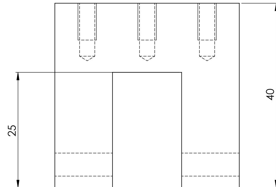
Vue Haut
