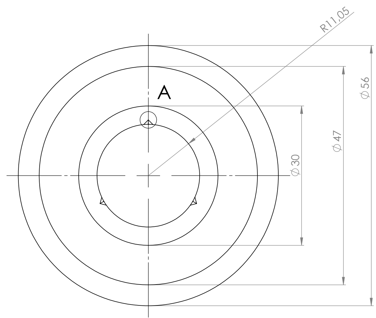
DÉTAIL A ECHELLE 10 : 1 Rainures lubrification 3x dépouilles 3°
