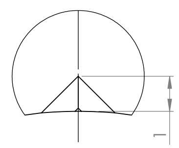
DÉTAIL A ECHELLE 10 : 1 Rainures lubrification 3x dépouilles 3°
