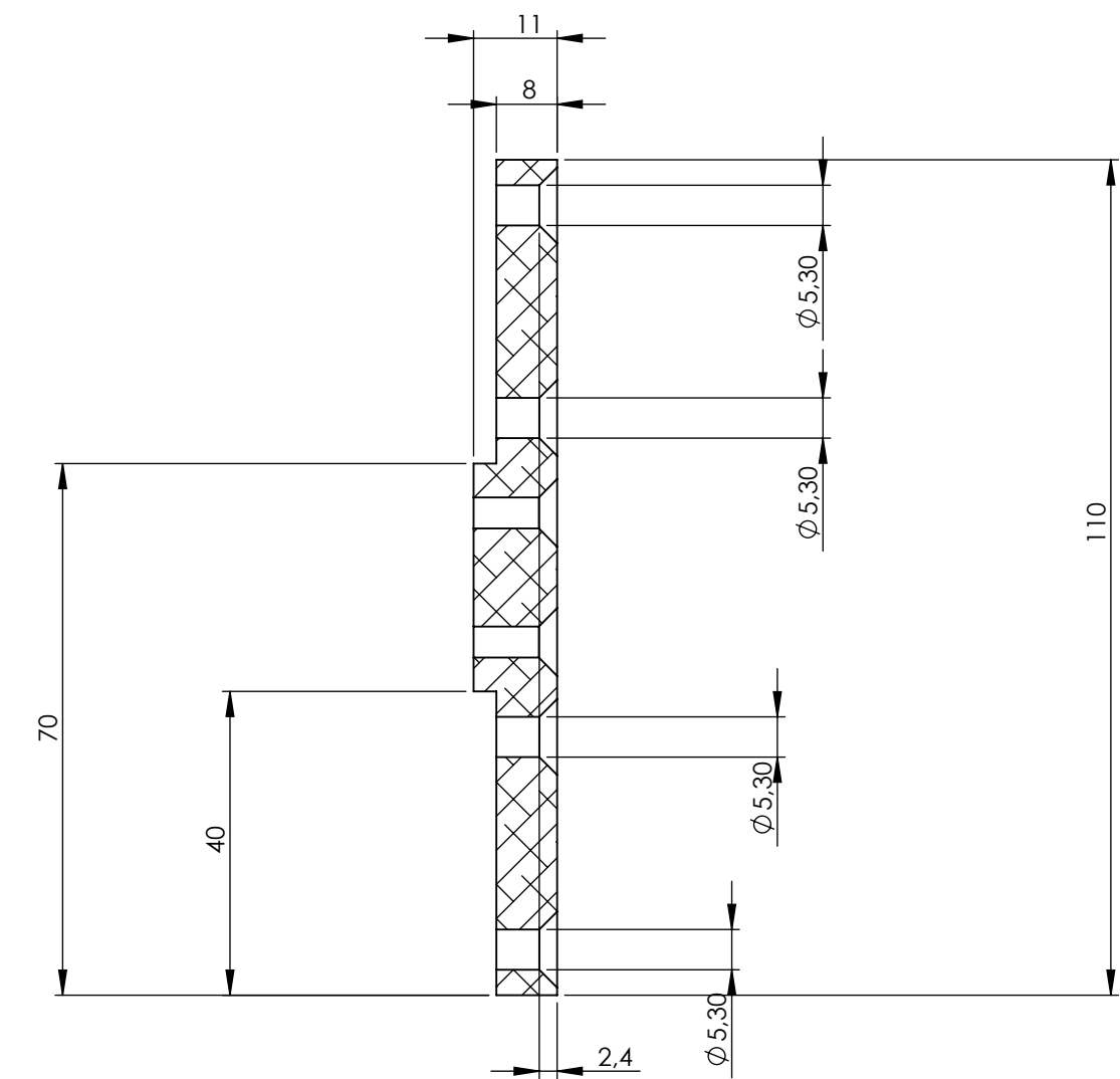
COUPE A-A
