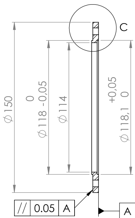
COUPE A-A
