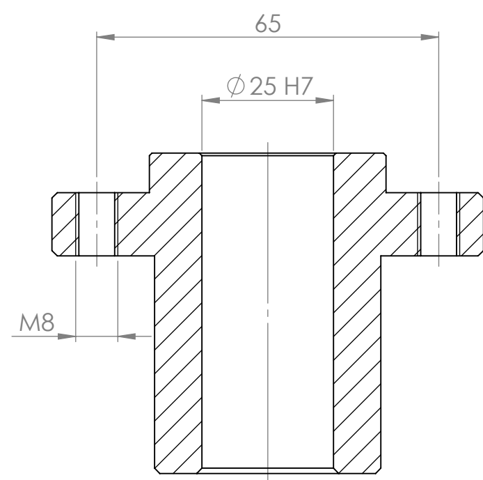
COUPE C-C ECHELLE 1 : 1
