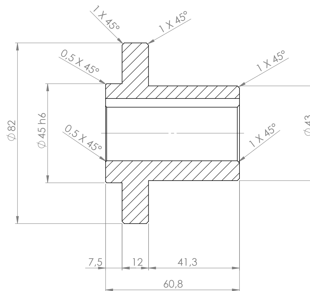
COUPE A-A ECHELLE 1 : 1
