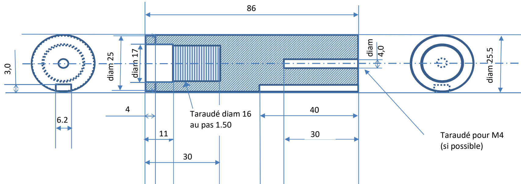
Coupe longitudinale
