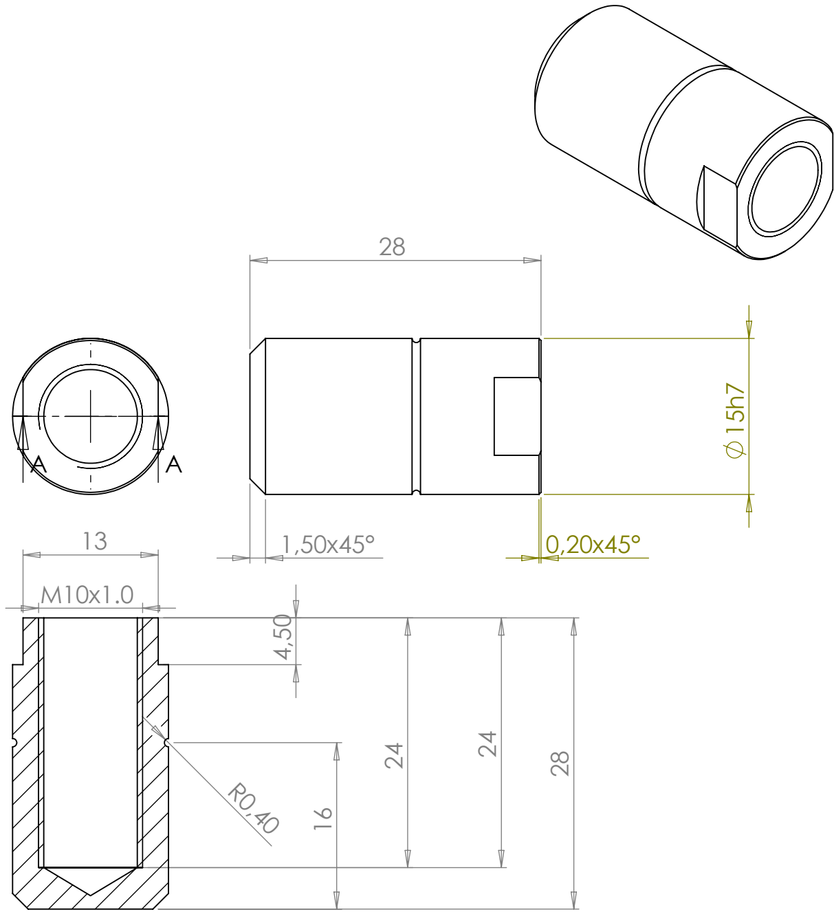
COUPE A-A
