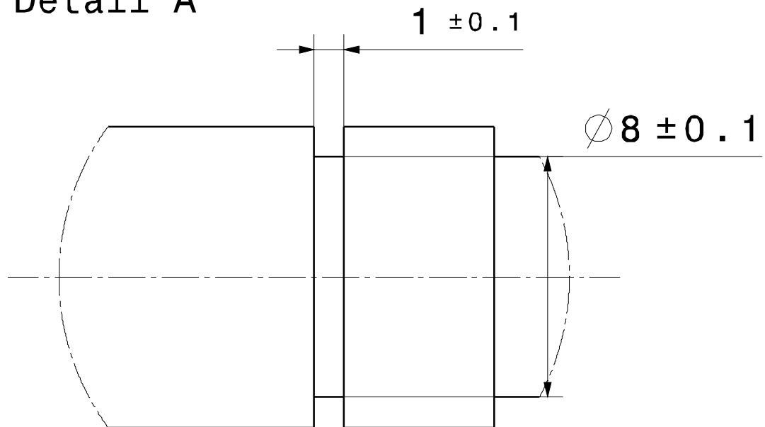
Détail A
