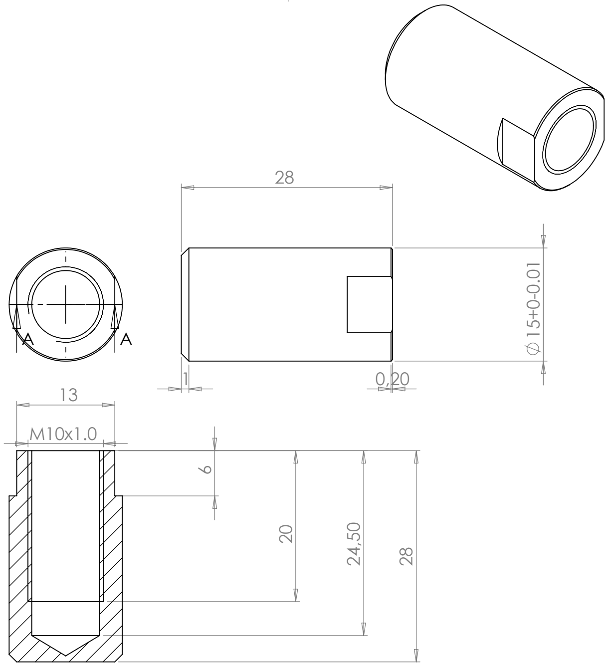
COUPE A-A
