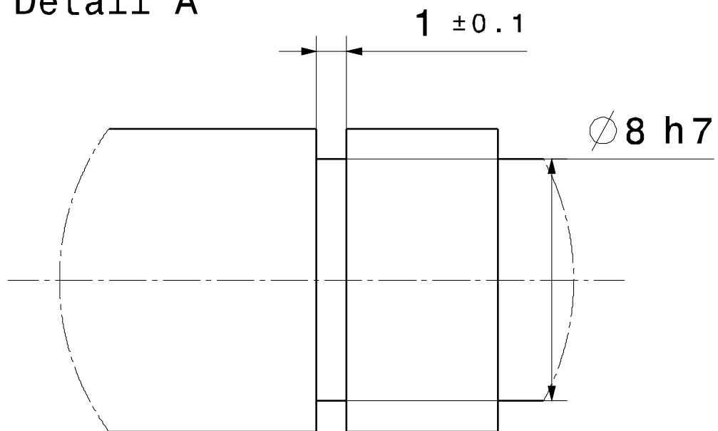
Détail A
