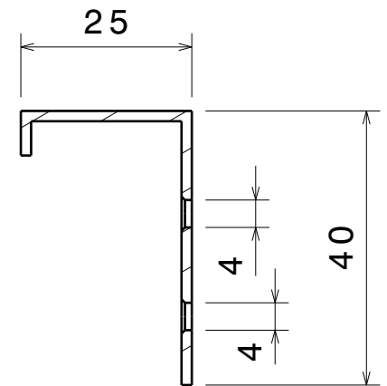
Coupe B-B Echelle : 1:1
