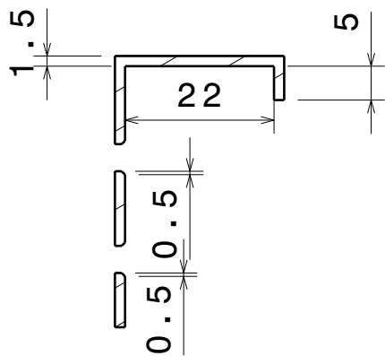
Section A-A Echelle : 1:1
