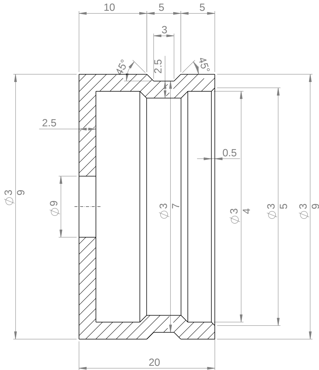
SECTION B-B SCALE 3 : 1
