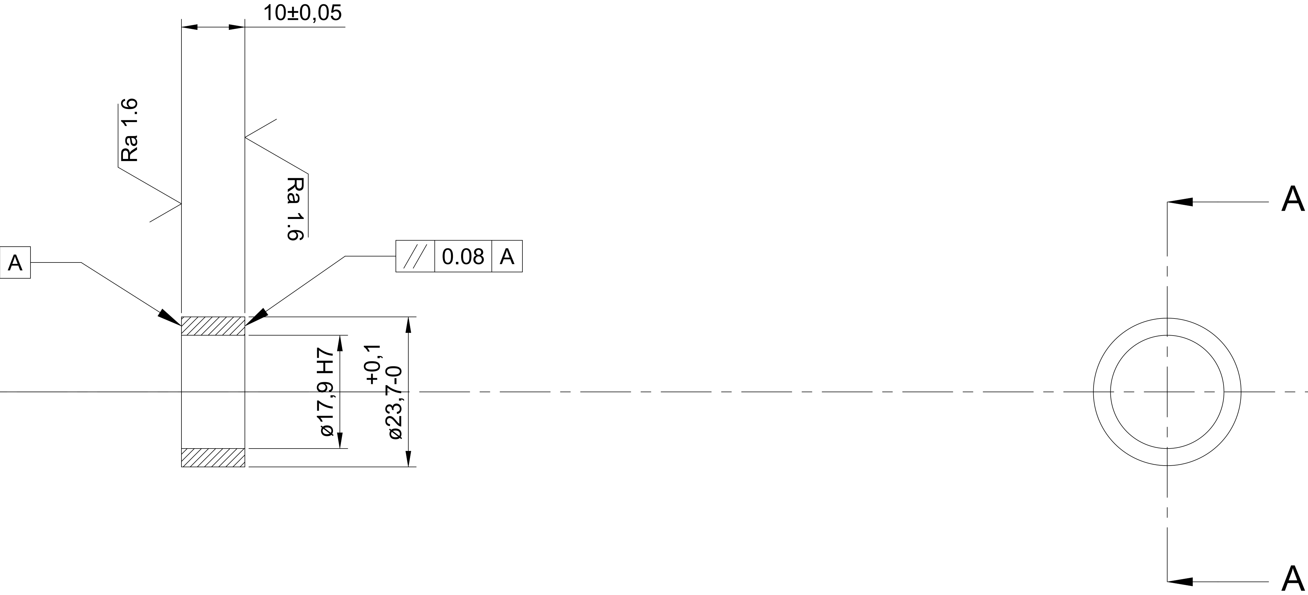
COUPE A-A
