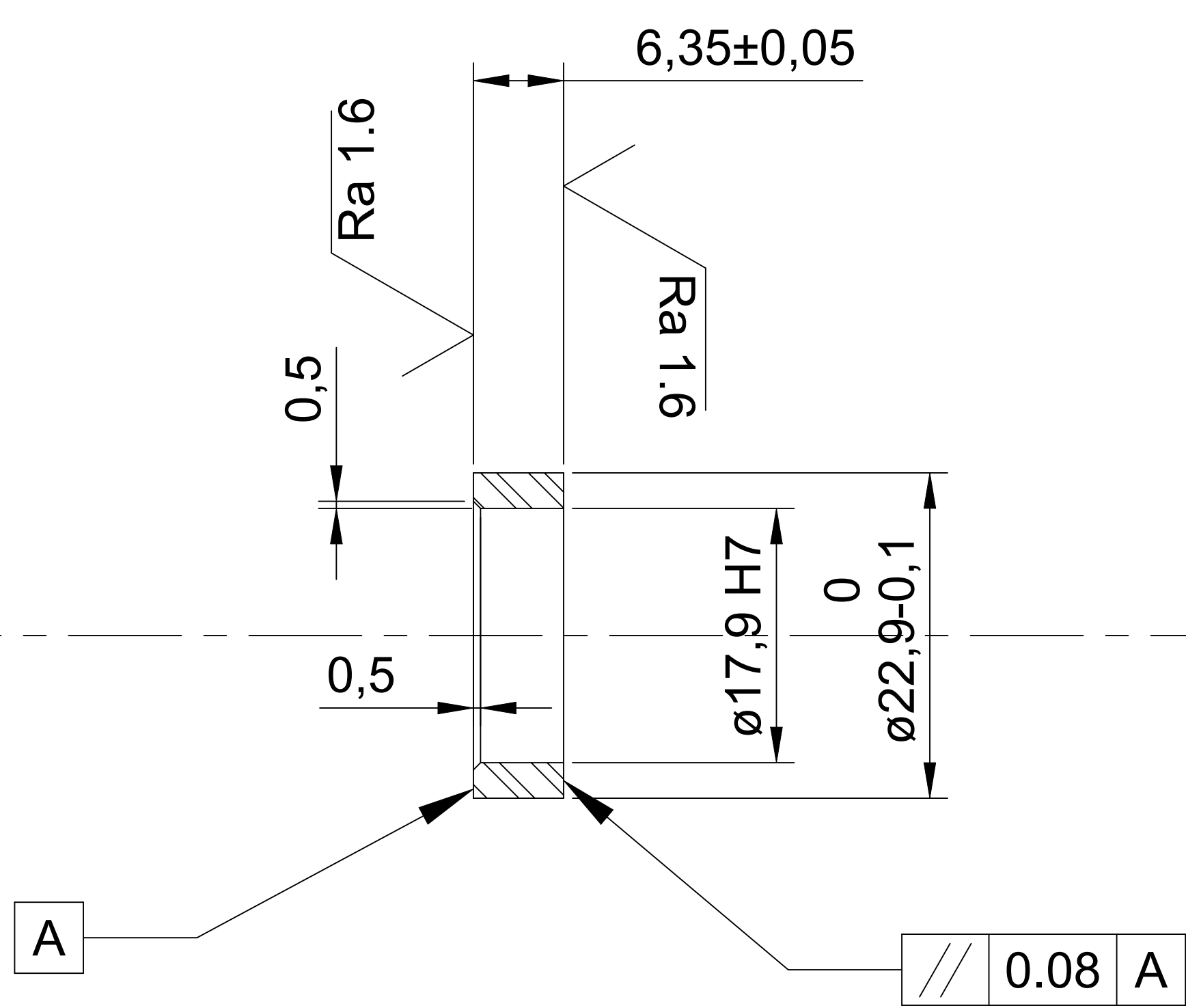
COUPE A-A
