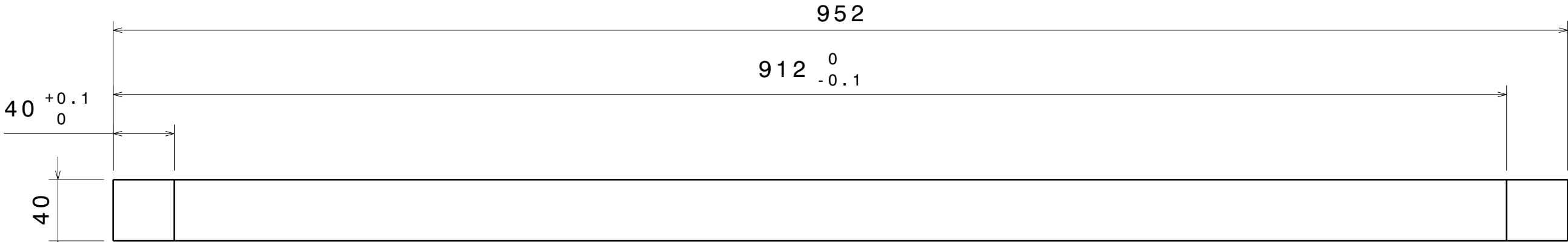
Vue de dessus Echelle : 1:3
