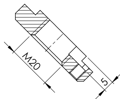
COUPE C-C
