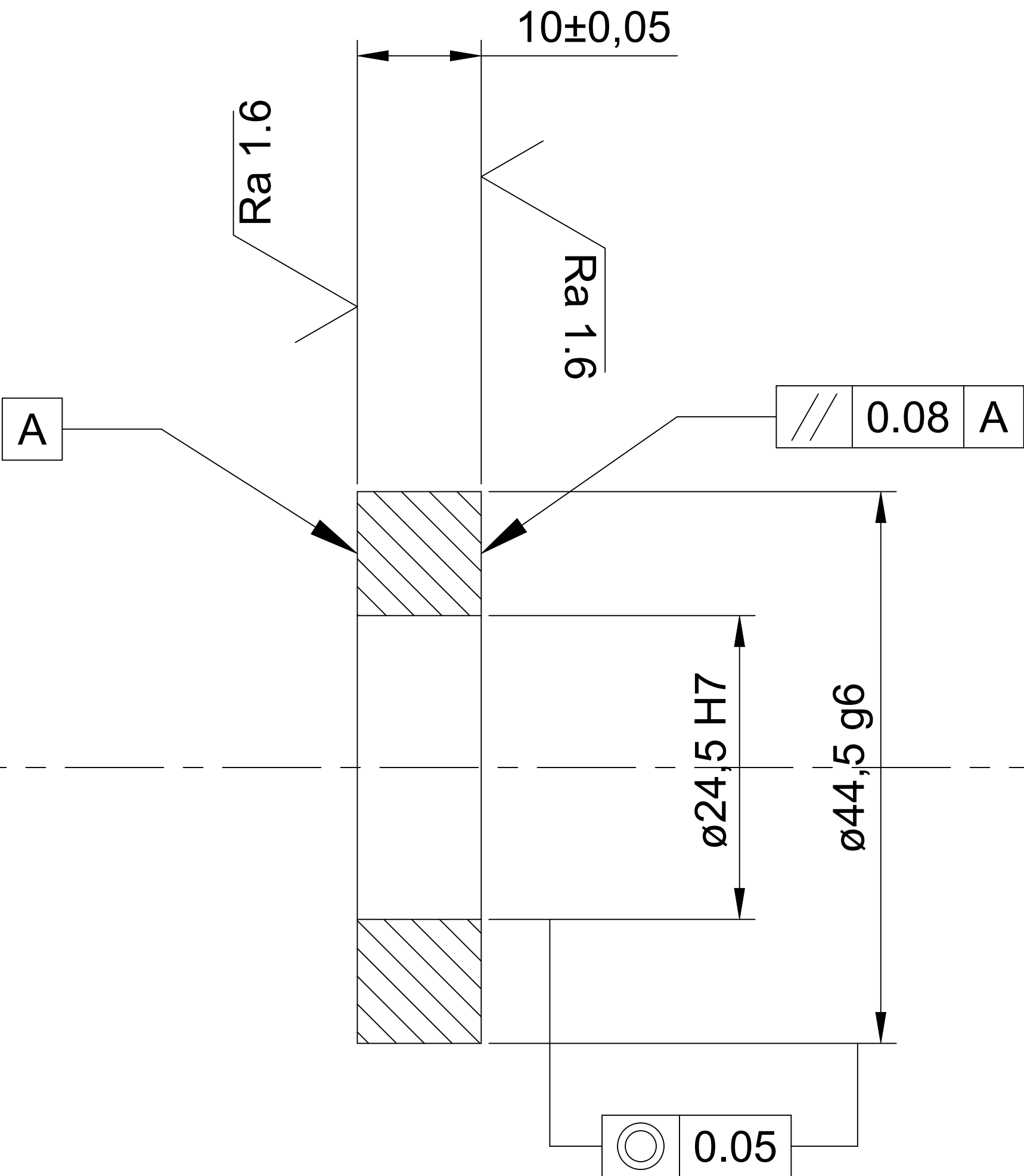
COUPE A-A
