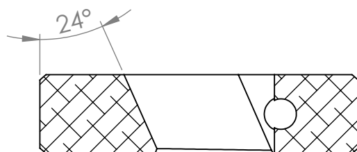
COUPE B-B ECHELLE 1 : 1
