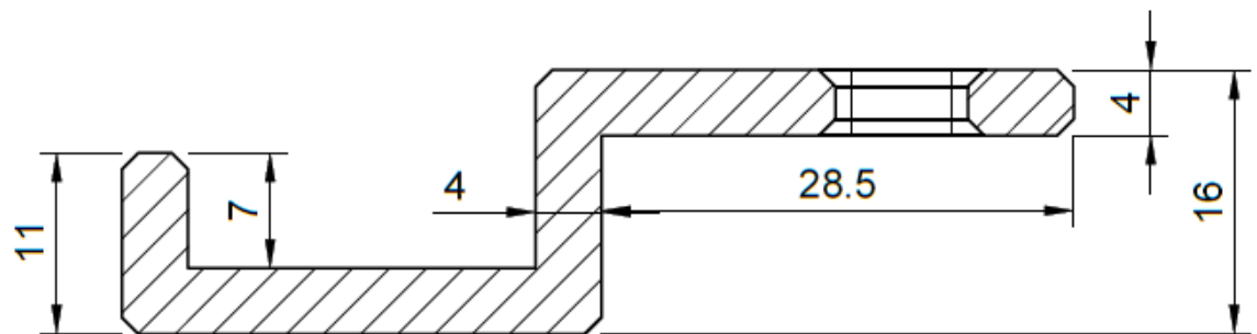
A-A (2:1)
